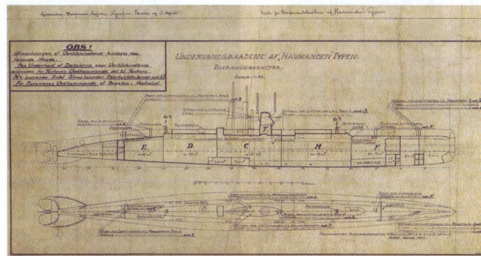
Bjergningsskitse fra Orlogsværftets konstruktionskontor for undervandsbåde af HAVMANDEN-klassen. Som det fremgår af artiklen kunne der meget vel været blevet brug for denne. (Forsvargalleriet)
